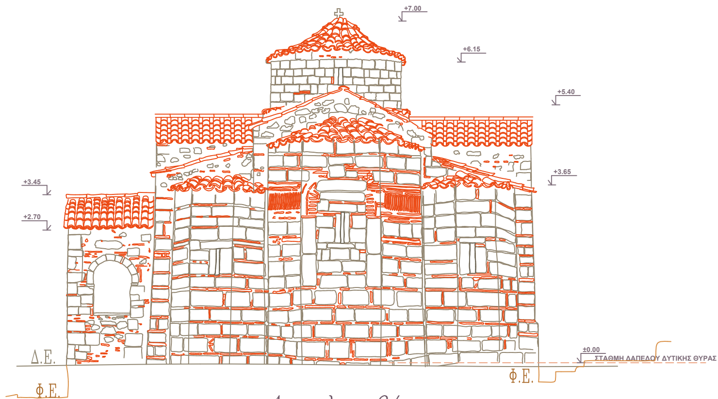
Ανατολική Οψη
